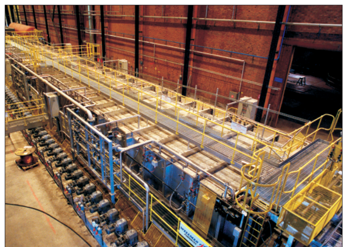
Bild 2: Rollenherdofen mit mehrstufiger Oxyfuel-Verbrennung
