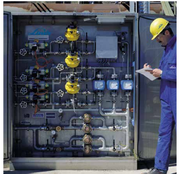
Gas-Dosiereinheit
