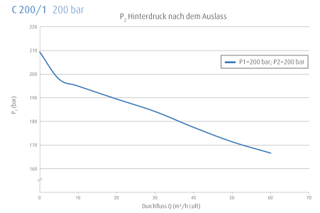
C 200/1 200 bar
